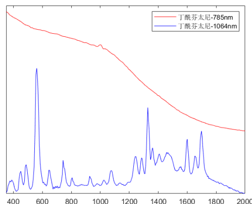
1064 nm激光波长可有效降低荧光干扰
