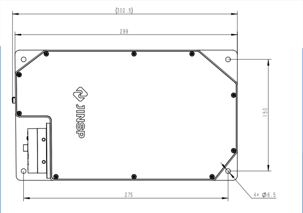
俯视图 (安装定位孔)
